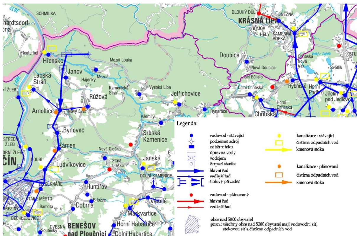
Obr. 4.1 Plán rozvoje vodovodů a kanalizací, zdroj: Plánu rozvoje vodovodů a kanalizací území České republiky
